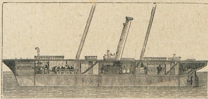
Coupe du « Saint-Michel ».
